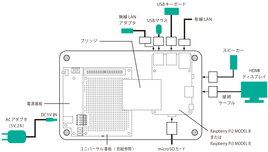
図 3.1.4 Rabyy Creator と周辺機器との接続図
